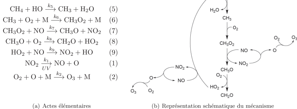
FIGURE 5 – Mécanisme simplifié de la production de l’ozone \text{O}_3 par le méthane.
