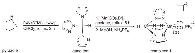
SCHEMA 1 – Synthèse du complexe 1
