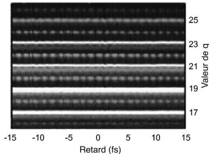
FIGURE 4 – Nombre de photoélectrons d'énergie E_q - I_P en fonction du retard \tau et de q , les zones les plus claires correspondant aux plus grands nombres [extrait de l'article “Physics of attosecond pulses produced via high harmonic generation”, par Katalin Varjú, Per Johnsson, Johan Mauritsson, Anne L’Huillier, Rodrigo López-Martens, Am. J. Phys. 77, 389–395 (2009)].
