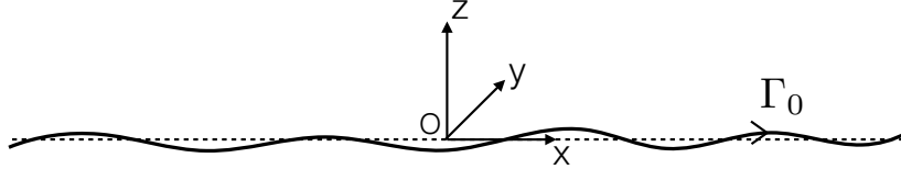
Figure 7: Une ligne de vorticité de circulation \Gamma déformée au voisinage de l'axe ( Ox ). En toute abscisse x , on note Y(x, t) et Z(x, t) les déformations transverses de la ligne par rapport à l'axe ( Ox ).
