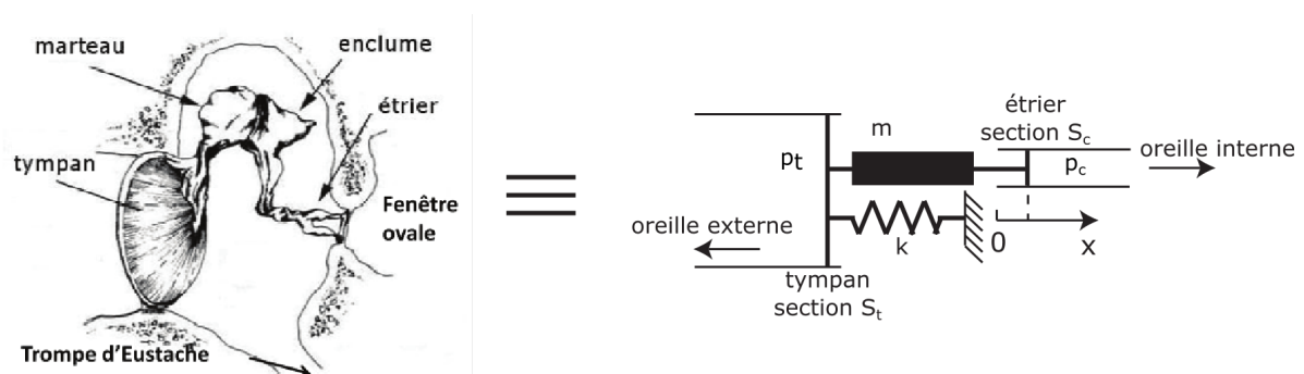
FIGURE 3 – On modélise l'oreille moyenne (à gauche) par un système masse-ressort qui relie rigidement un piston du côté de l'oreille externe de section S_t à un autre piston du côté de l'oreille interne de section S_c . On note x(t) l'abscisse de ce second piston à l'instant t .
