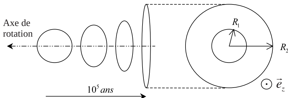
Figure 2 : Aplatissement d'une nébuleuse initialement sphérique sous l'effet de sa rotation propre. Vue de dessus de sa modélisation par un tore.
