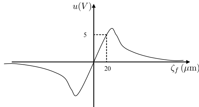
Figure 13 : Courbe de réponse de la mesure de défocalisation par senseur astigmatique : \zeta_f représente le décalage, dans le sens du rayon laser, entre la position effective du disque et celle du spot focalisé ; en régime linéaire, la tension u aux bornes du détecteur est proportionnelle à \zeta_f .
