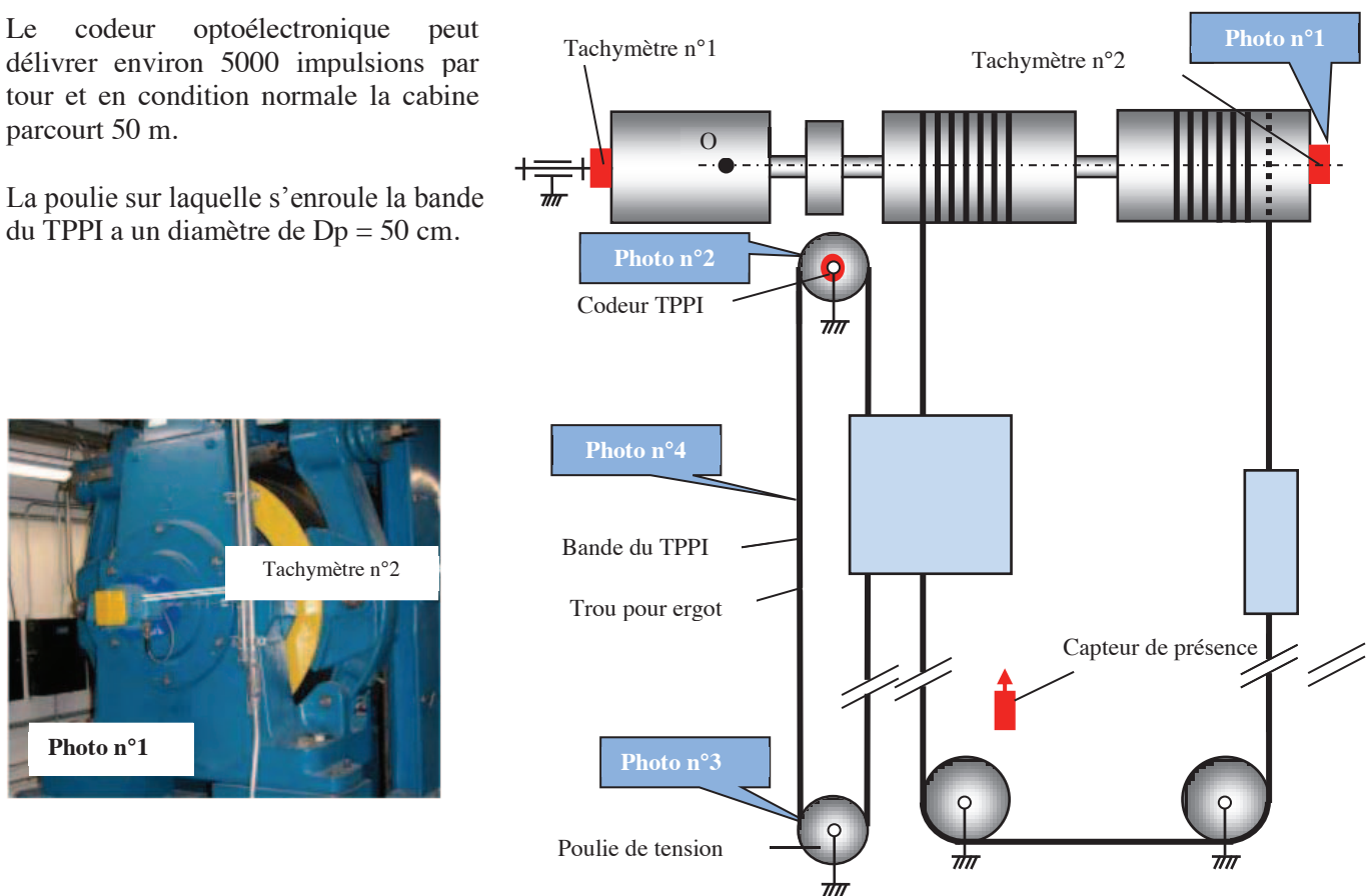
Fig. 11 : mesure de la position de la cabine
