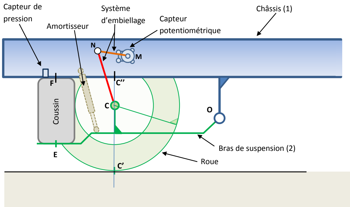
Vue schématique d'un essieu équipé d'une suspension pneumatique ECS
