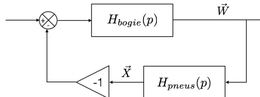
Figure 20 : schéma d'asservissement caractéristique du phénomène de shimmy
