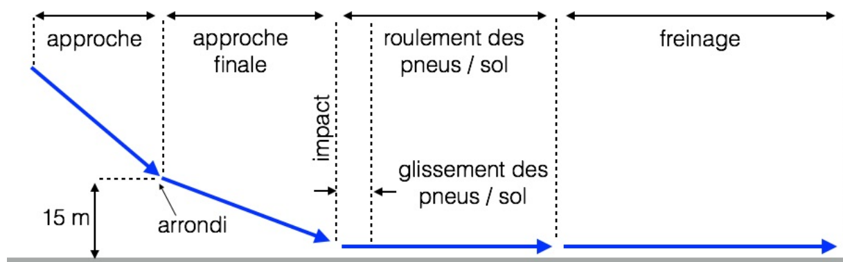
Figure 2 : chemin de vol de l'avion en phase d'atterrissage
